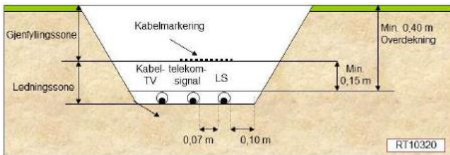
Figur RT10320: Hovedprinsipp ved forlegning av kabelstikkledning \leq 95\text{mm}^2 på privat grunn
