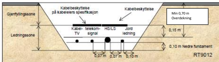
Figur RT9012: Hovedprinsipp ved forlegning av lavspent stikkledning > 95\text{mm}^2 samt kabler utenfor privat grunn
